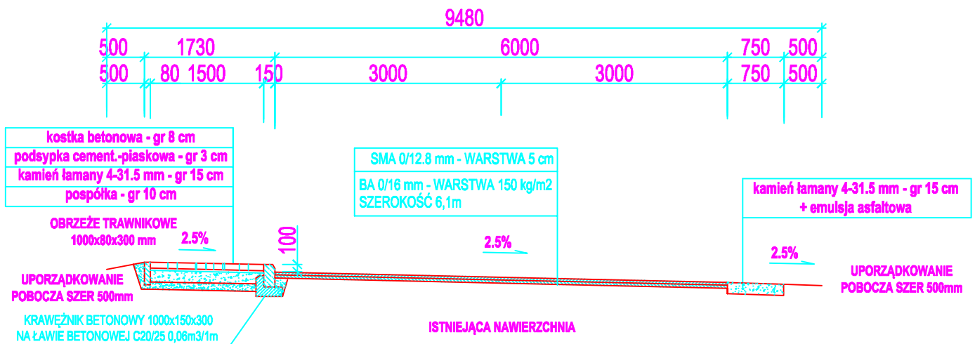
PRZEKRÓJ KONSTRUKCYJNY - PRZEBIEG Z CHODNIKIEM - (km 1+290)
