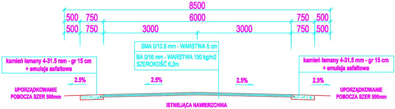
PRZEKRÓJ KONSTRUKCYJNY - PRZEBIEG BEZ CHODNIKA - (km 0+100)
