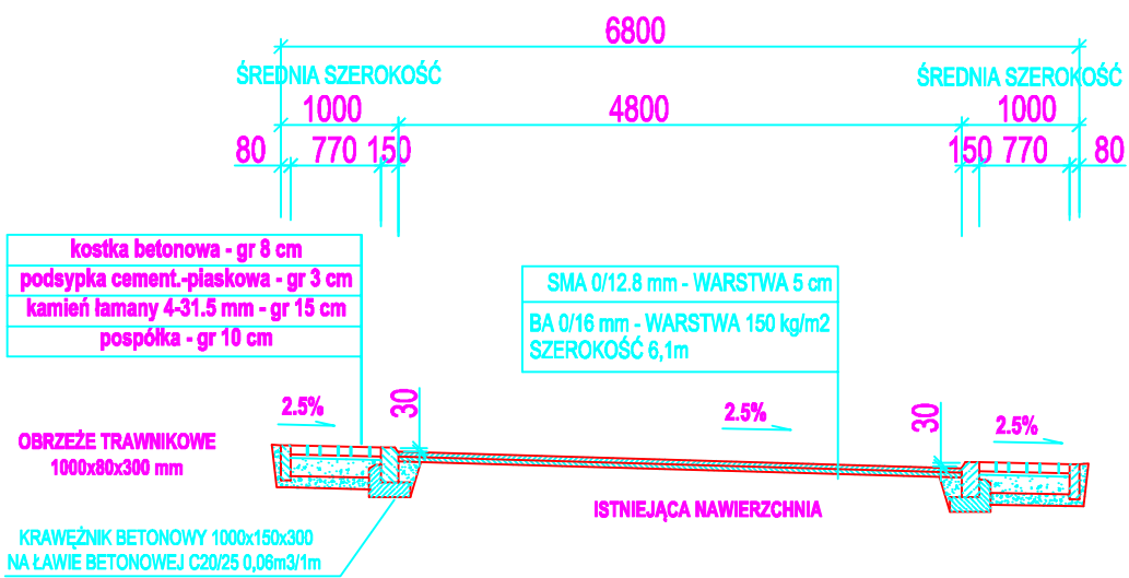
PRZEKRÓJ KONSTRUKCYJNY - (km 0+100)
