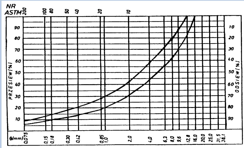
Rys. 3. Krzywe graniczne uziarnienia mieszanki mineralnej 0÷16 mm do warstwy ściaralnej z betonu asfaltowego dla KR 3-6
